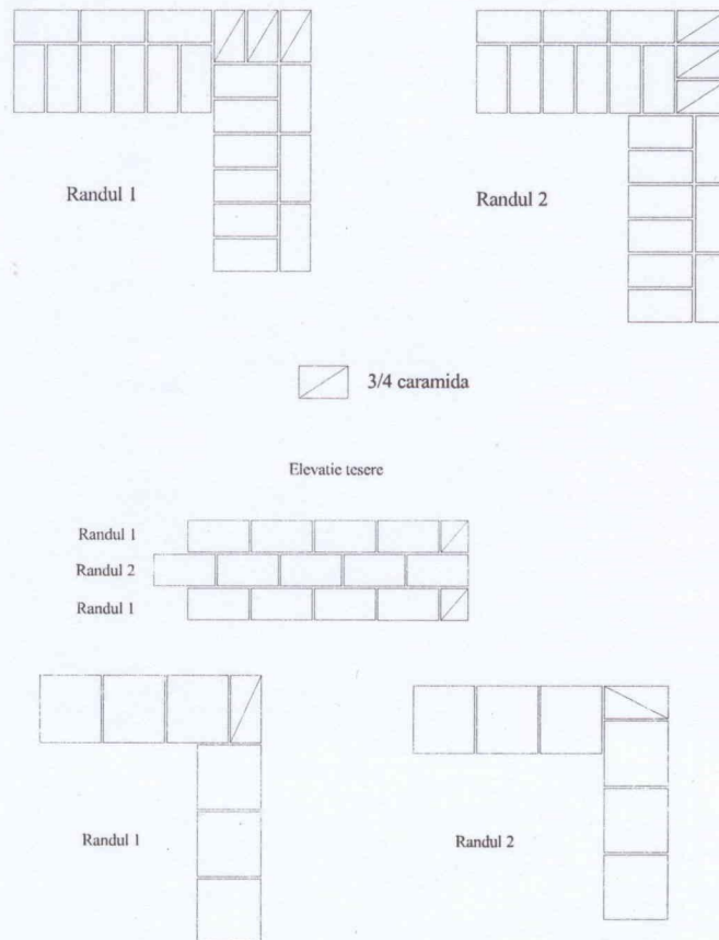
Figura 3. Legături la colțuri pentru elemente de zidărie cu înălțime de asiza \leq 150\text{mm}
