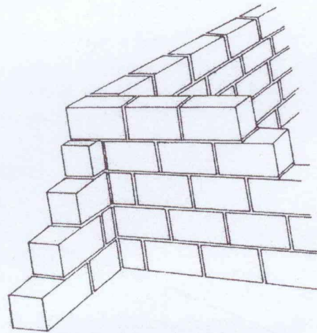
Figura 8. Țeserea zidăriei din BCA în trepte la colțuri, fără stâlpișor de confinare
