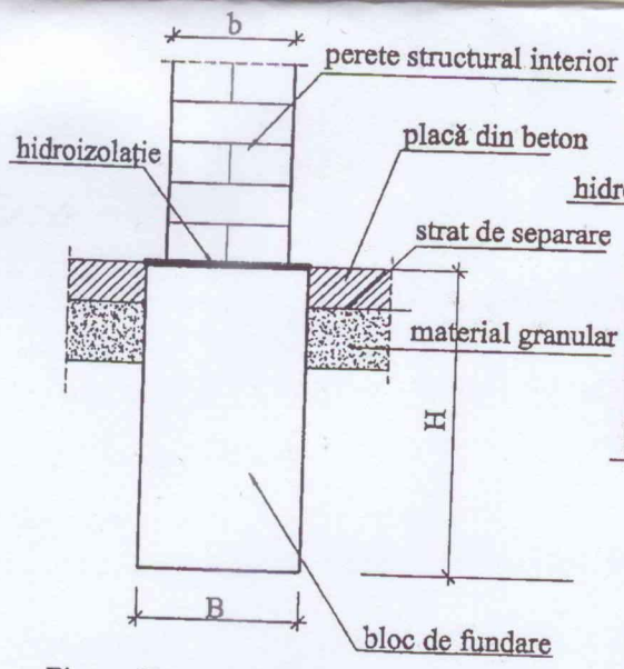
Figura II.22.a – Bloc de fundație din beton simplu
