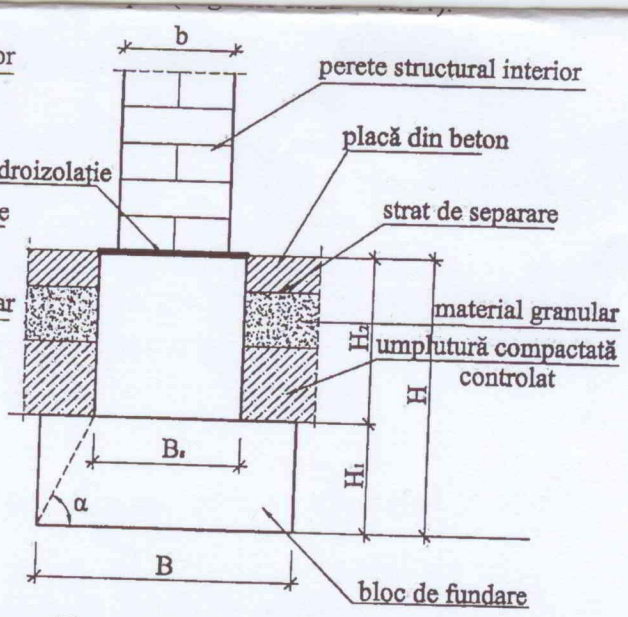
Figura II.22.b - Bloc de fundație și soclu din beton simplu
