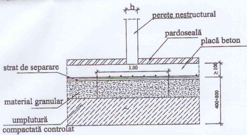
Figura II.35 - Armare suplimentară locală a plăcii pe sol pentru susținerea unui perete nestructural
