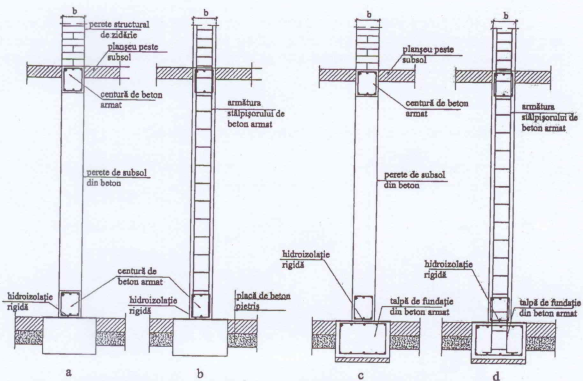
Figura II.26 - Pereți de subsol din beton simplu cu centuri din beton armat la extremități, tălpi de fundații din beton simplu (a și b) și tălpi din beton armat (c și d)
