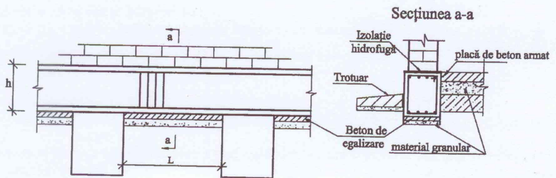
Figura II.30 - Fundații cu descărcări pe reazeme izolate
