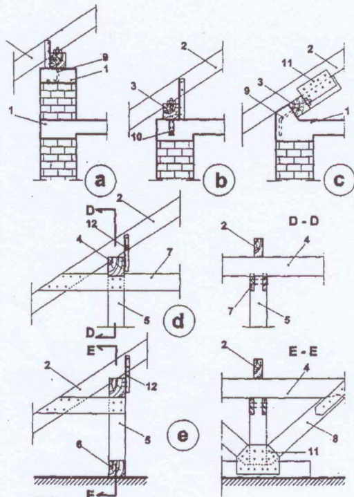
FIG. R2 DETALI DE SARPANTE DIN LEAM PE SCAUNE
