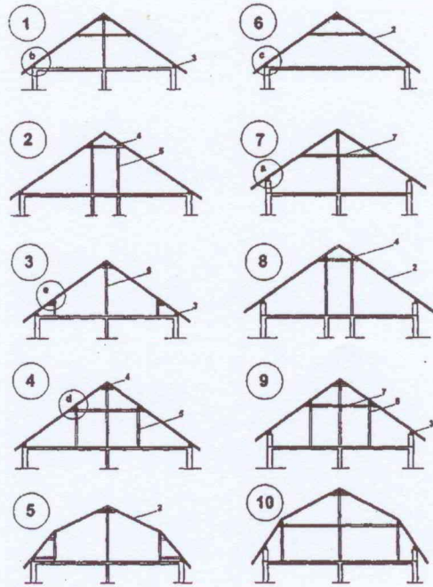
FIG. R1 EXEMPLE DE SARPANTE DIN LEAM PE SCAUNE
