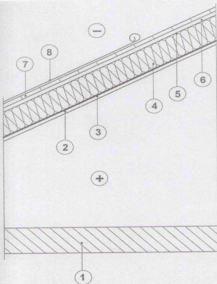
Fig. 11 Acoperiș cu pod mansardat. Izolație termică între căpriori (soluție de principiu)
