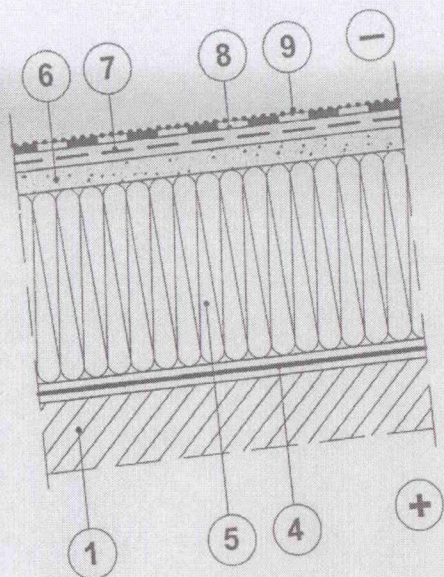
Fig. 3 Acoperiș cu alcătuire compactă cu planșeu inclinat (soluție de principiu)
