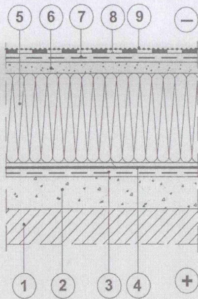
Fig. 4 Acoperiș cu alcătuire compactă cu planșeu orizontal și beton de pantă (soluție de principiu)
