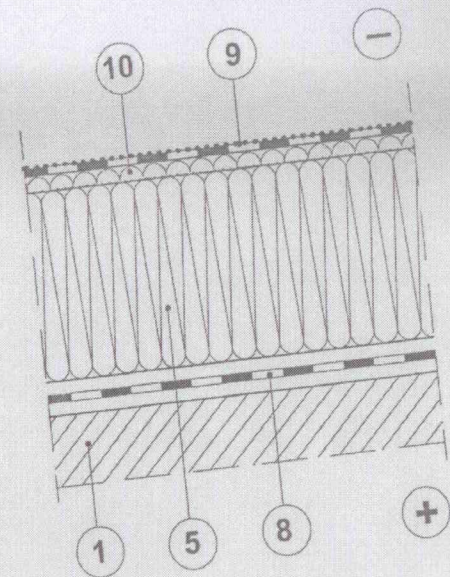
Fig. 5 Acoperiș cu alcătuire compactă cu invelitoare inversă / ranversată (soluție de principiu)
