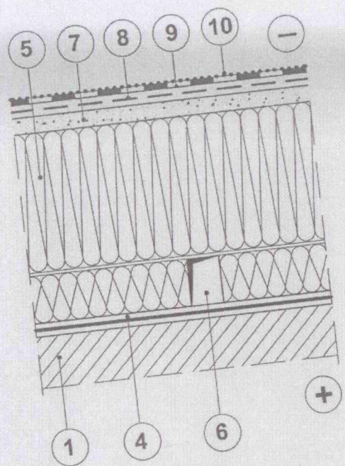
Fig.6 Acoperiș cu alcătuire ventilată cu planșeu înclinat (soluție de principiu)
