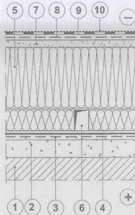
Fig.7 Acoperiș cu alcătuire ventilată cu planșeu orizontal cu beton de pantă (soluție de principiu)
