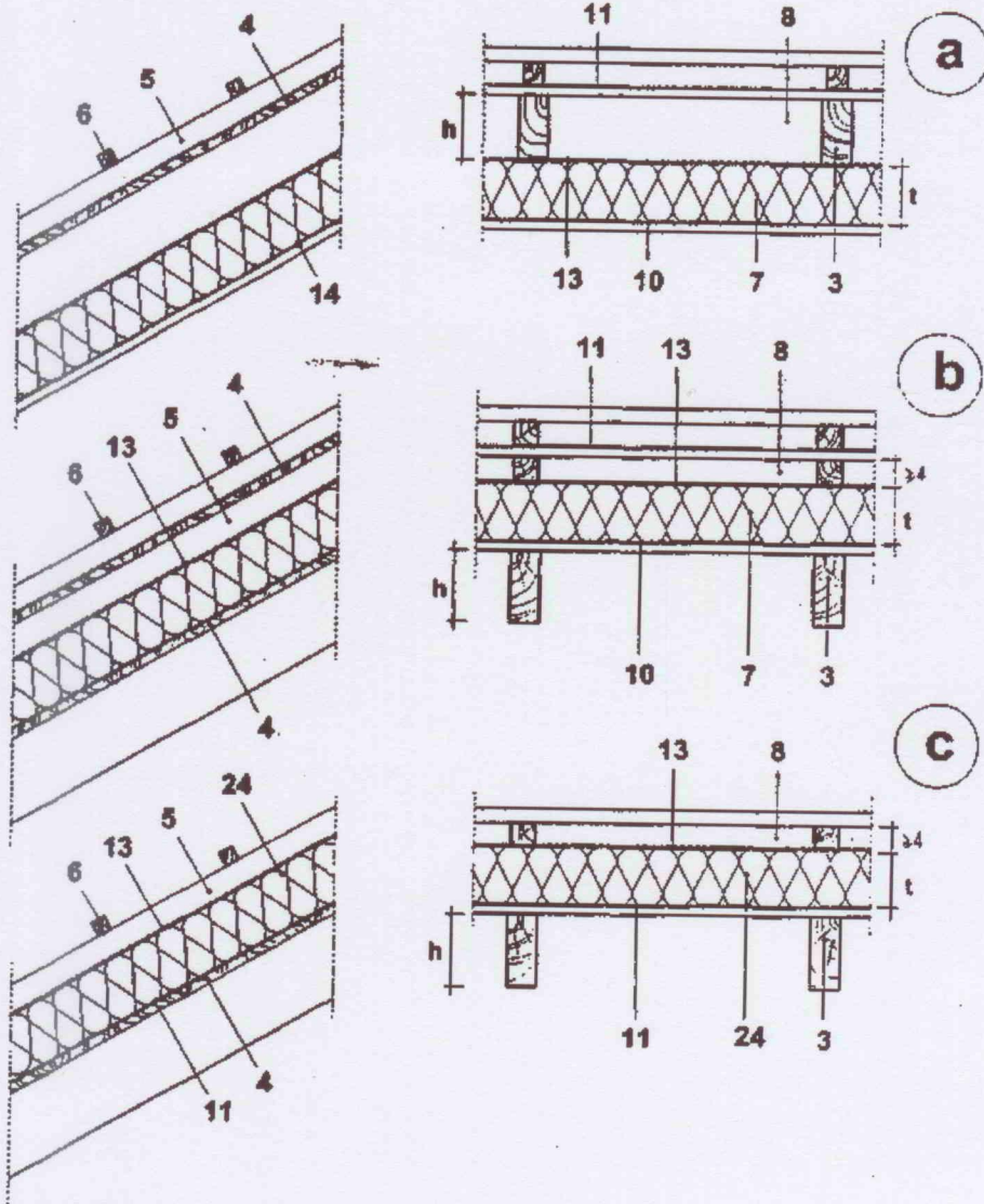
FIG. 14 AMPLASAREA STRATULUI TERMORIZANT SUB SAU PESTE CAPRIORI
