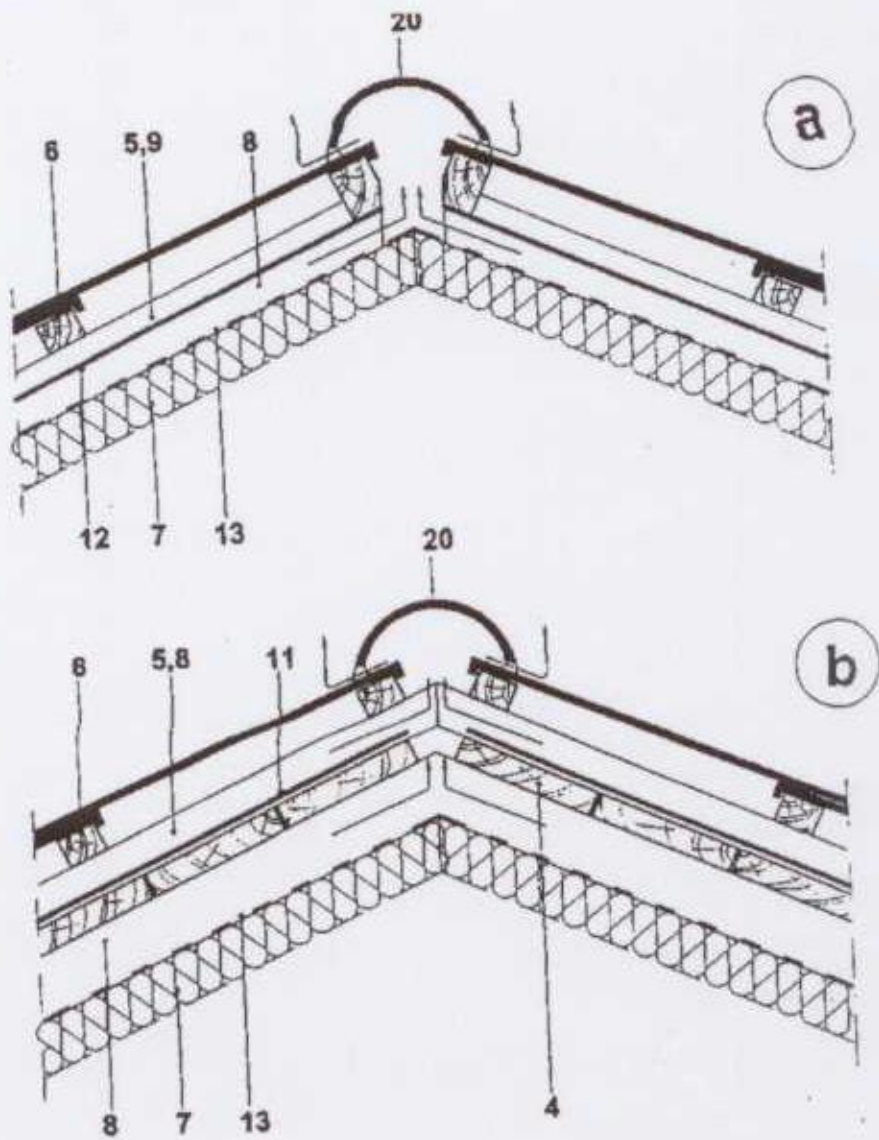
FIG. T10 DETALII LA COAMA a. CU UN STRAT DE AER VENTILAT b. CU DOUA STRATURI DE AER VENTILAT
